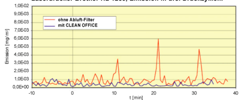
Vergleich der Feinstaub-Emission MIT und OHNE Staubfilter: Laserdrucker Brother HL 1250, Emission in drei Druckzyklen.
